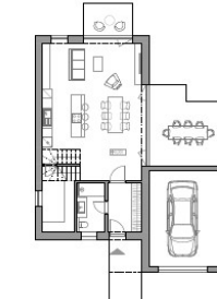
PODORYS 1.NP
