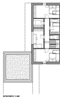
PODORYS 2.NP
